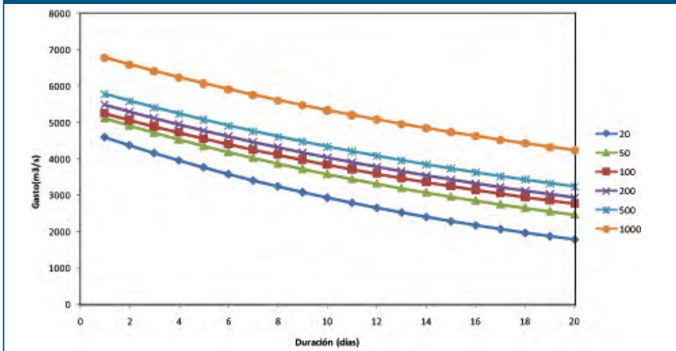
Figura 10. Curvas de reducción de los gastos promedio para diferentes duraciones y periodos de retorno
