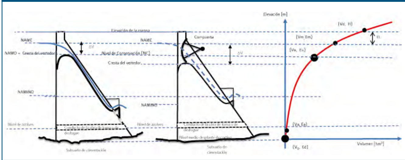
Figura 2. Curva elevaciones-capacidades del tertedor. Representación gráfica de los volúmenes de almacenamiento de agua respecto a las elevaciones topográficas del embalse
