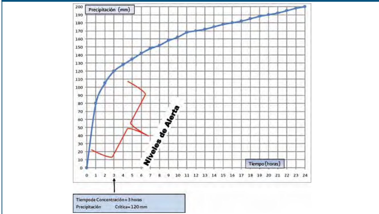
Figura 8. Precipitación acumulada para una tormenta de período de retorno de 2 años
