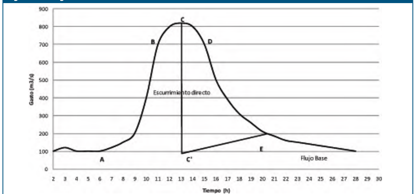
Figura 4. Hidrograma de escurrimiento
