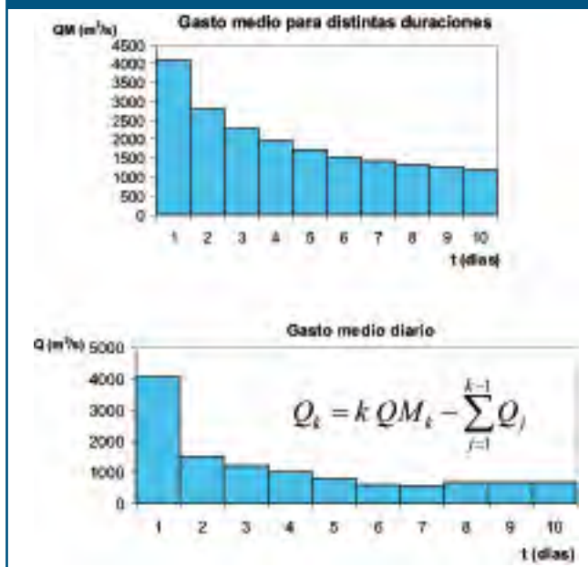
Figura 11. Cálculo de gastos medios diarios Q_k
