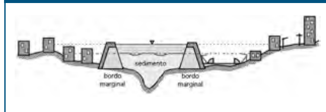
Figura 3.3. Cauce con bordos que ya se ha sedimentado
