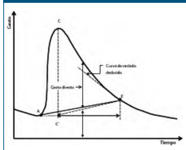
Figura 7. Separación del escurrimiento directo y base utilizando la curva de vaciado
