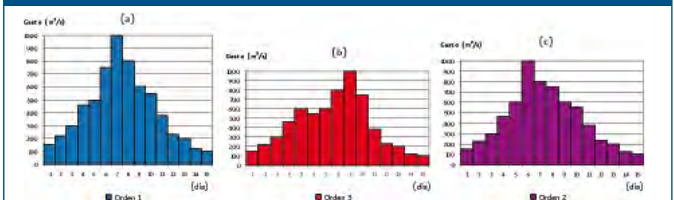
Figura 12. Alternativas de ordenamiento del hidrograma de diseño
