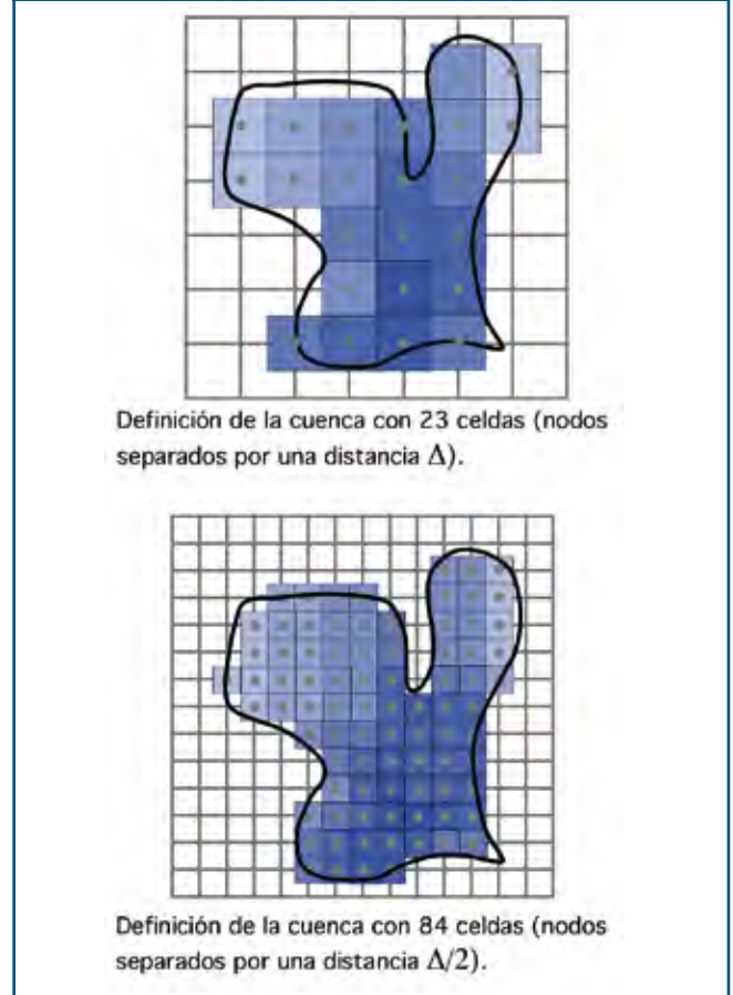
Figura 2.1.5. Mejor definición de la cuenca con malla más fina
