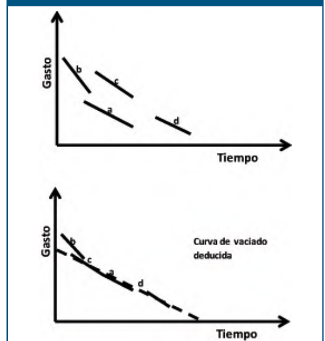
Figura 6. Curva de vaciado de diferentes hidrogramas
