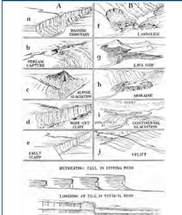
Figura 3. Tipo de cascadas que se desarrollan en las cuencas altas
