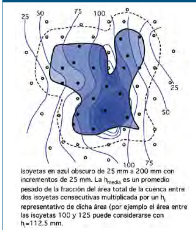
Figura 2.1.3. Método de isoyetas
