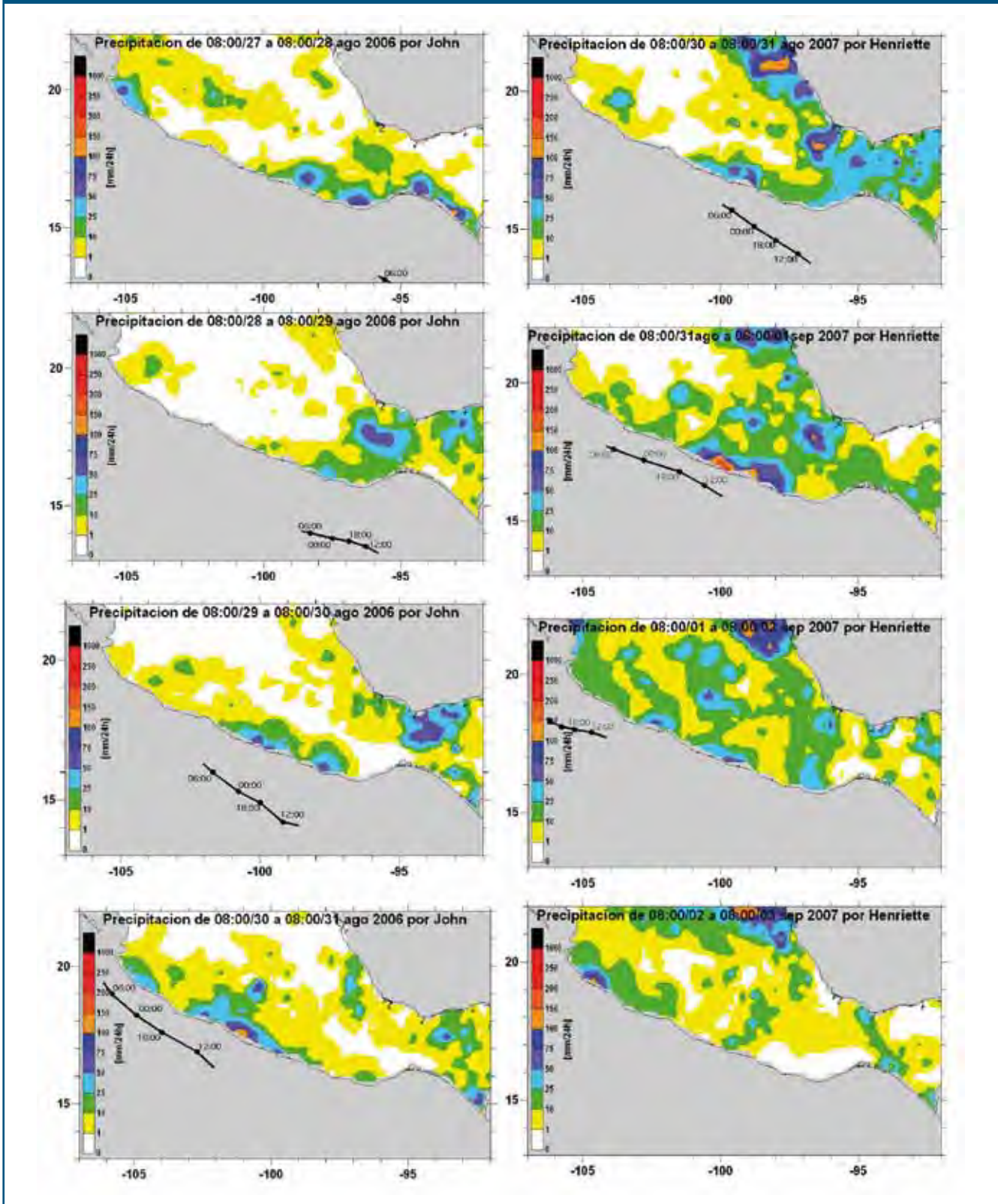
Figura 8. Evolución de las huellas de precipitación generada por ciclones tropicales con trayectorias pseudo paralelas a la costa Pacífico Sur de México (John, 2006 y Henriette, 2007). Observe la tendencia de las mayores acumulaciones por detrás de la trayectoria recorrida en cada día
