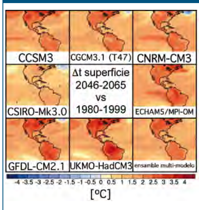
Figura 6. Comparación de incrementos proyectados por ocho modelos globales y el ensamble para la temperatura del aire en la superficie en la vecindad de México con un horizonte del orden de 50 años
