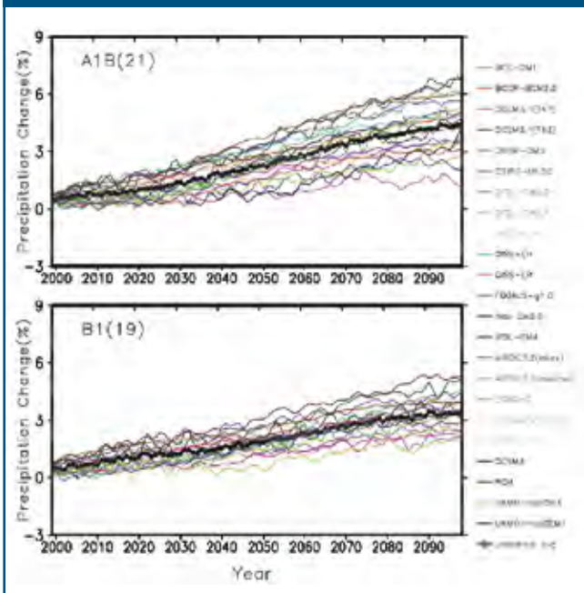
Figura 5. Evolución del cambio en la precipitación promedio global proyectada por 21 y 19 modelos distintos para dos escenarios (A1B y B1) moderados del IPCC (Fuente: IPCC, 2007, Fig.10.5)
