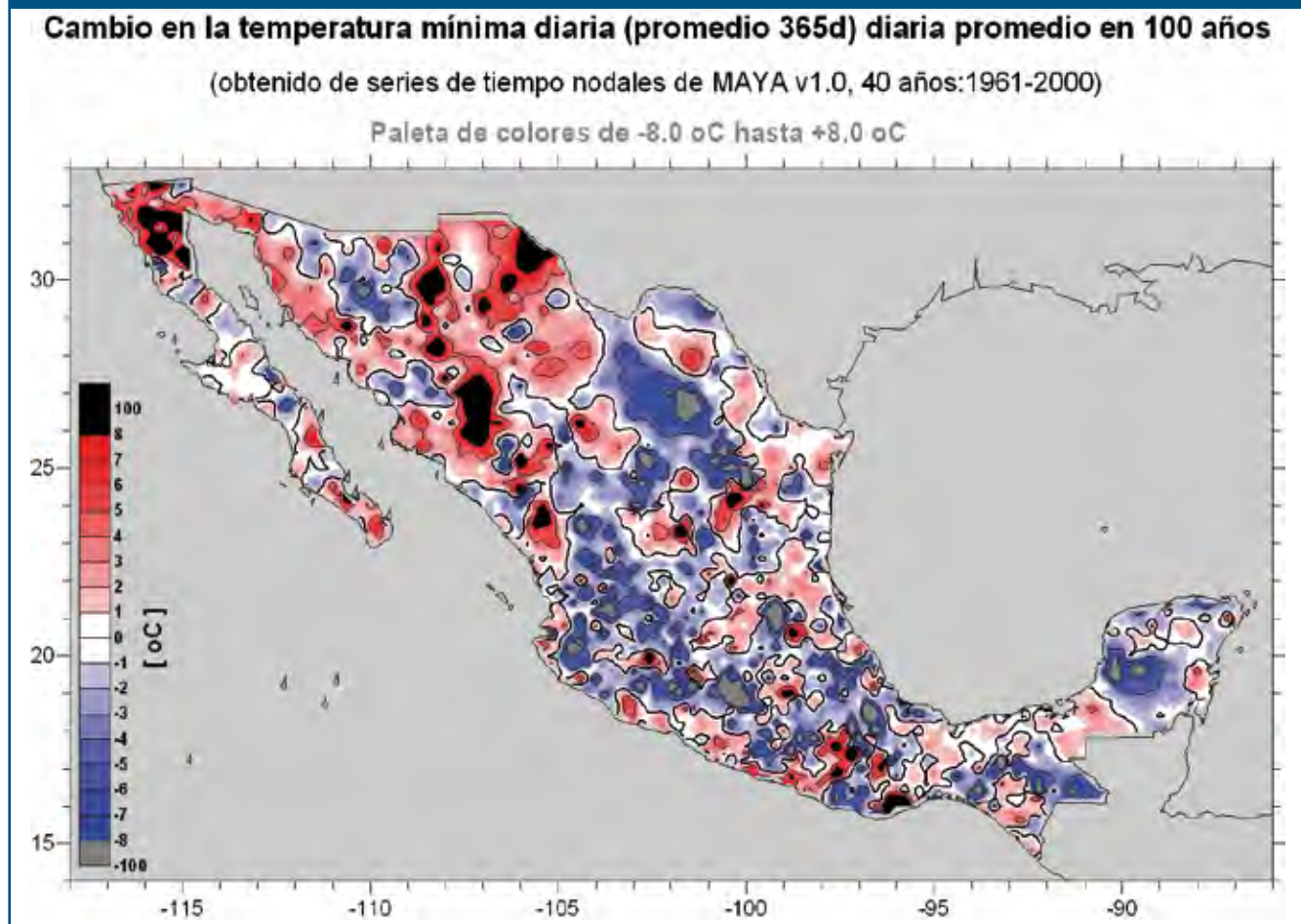
Figura 12. Distribución espacial de la tendencia de T_{min} observada desde 1961 a 2000
