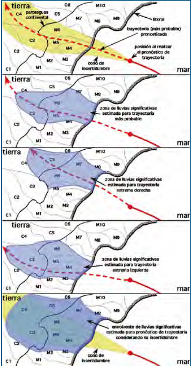
Figura 9. En el panel superior se muestra una trayectoria pronosticada con su cono de incertidumbre. En los siguientes tres paneles se muestran las zonas estimadas con lluvias significativas para la trayectoria más probable (central), la trayectoria extrema derecha y la trayectoria extrema izquierda. En el panel inferior se muestra la envolvente de las tres zonas previas, la adecuada para la toma de decisiones con la incertidumbre presente
