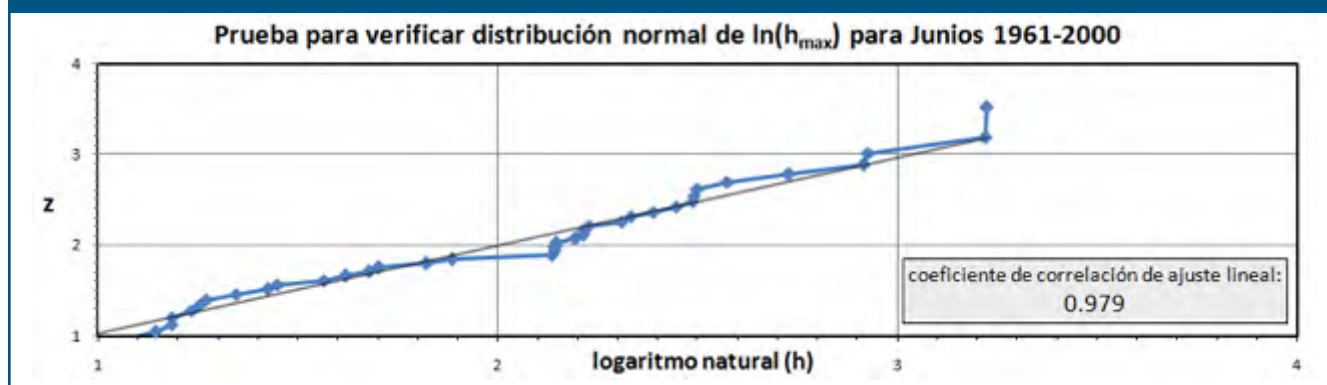
Figura 1.2.1.A- 3. Verificación de que la muestra de junio se ajusta bien a una distribución log-normal
