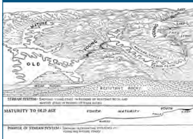
Figura 2. Etapas de desarrollo de un río en la cuenca media ( madure stream )
