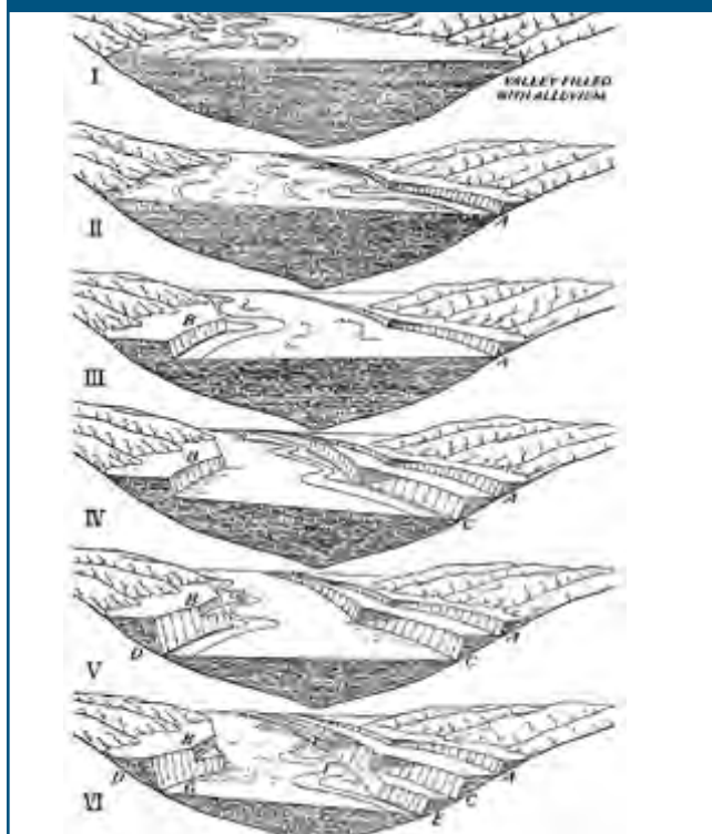
Figura 4. Formación de terrazas aluviales en un valle tipo "U", en una cuenca media
