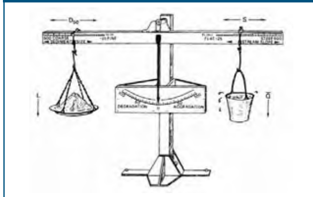
Figura 4. Balanza de Lane. Procesos naturales en el equilibrio dinámico de un sistema fluvial Q = Caudal, L = carga de sedimento, D_{50} tamaño medio del sedimento, S = pendiente hidráulica del cauce
