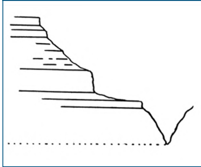
Figura 1. Sección tipo "V" de un cauce en cuenca alta
