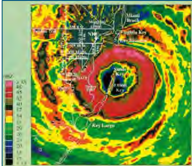
Figura 3. El huracán Andrew observado desde el radar ubicado en el Centro Nacional de Huracanes de los EUA el 24 de agosto de 1992. La extensión cubierta por la gráfica es de 100 km por 100 km. Se observa claramente la llamada pared del ojo
