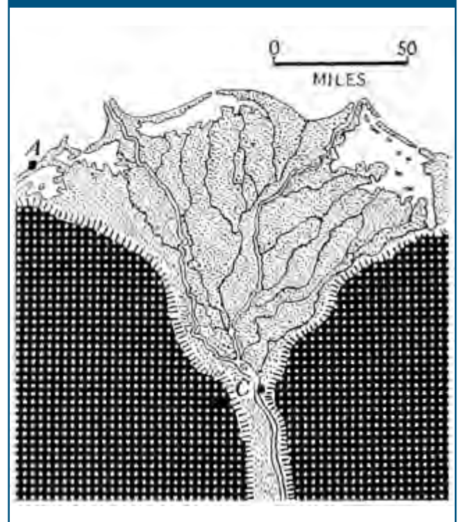
Figura 6. Desarrollo de un delta en zona de descarga de una cuenca baja
