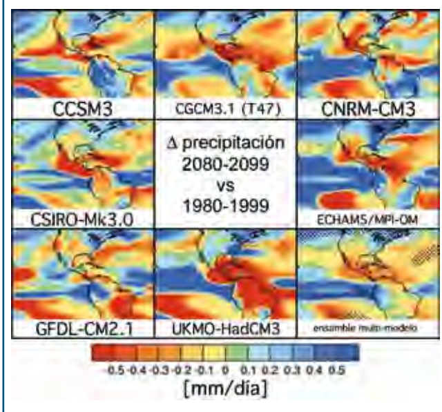
Figura 7. Comparación de cambios proyectados por ocho modelos globales y el ensamble para la precipitación pluvial en la vecindad de México con un horizonte del orden de 100 años
