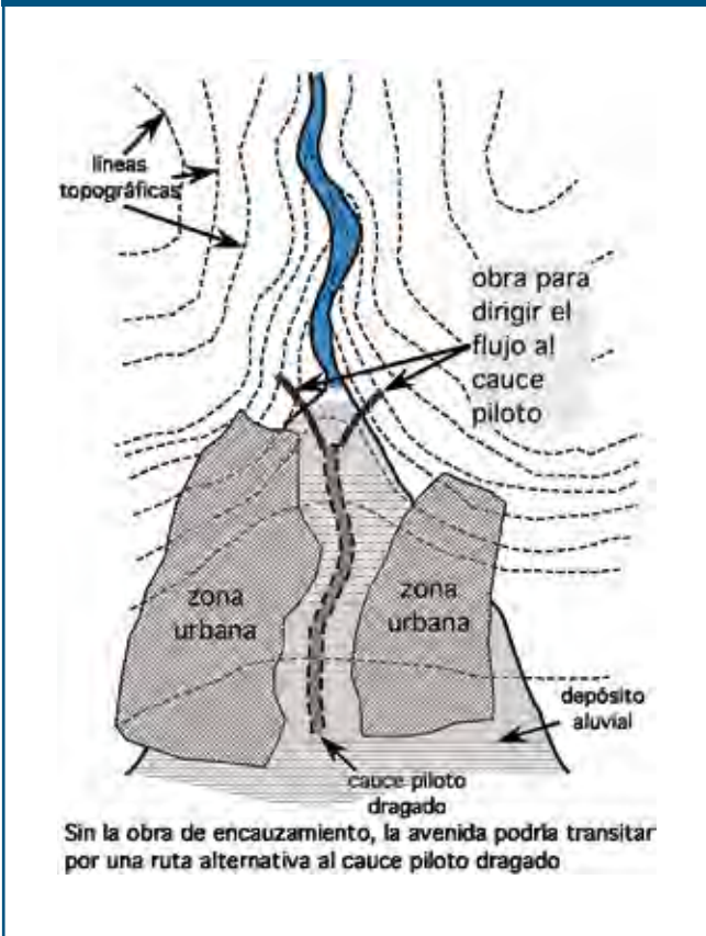
Figura 3.5. Obras de encauzamiento necesarias aguas arriba de un cauce piloto dragado
