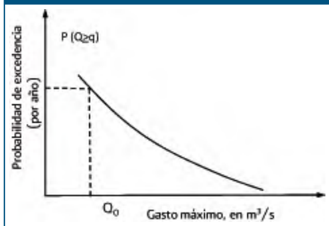
Figura 15. Q_{\text{diseño}} - Probabilidad de Excedencia
