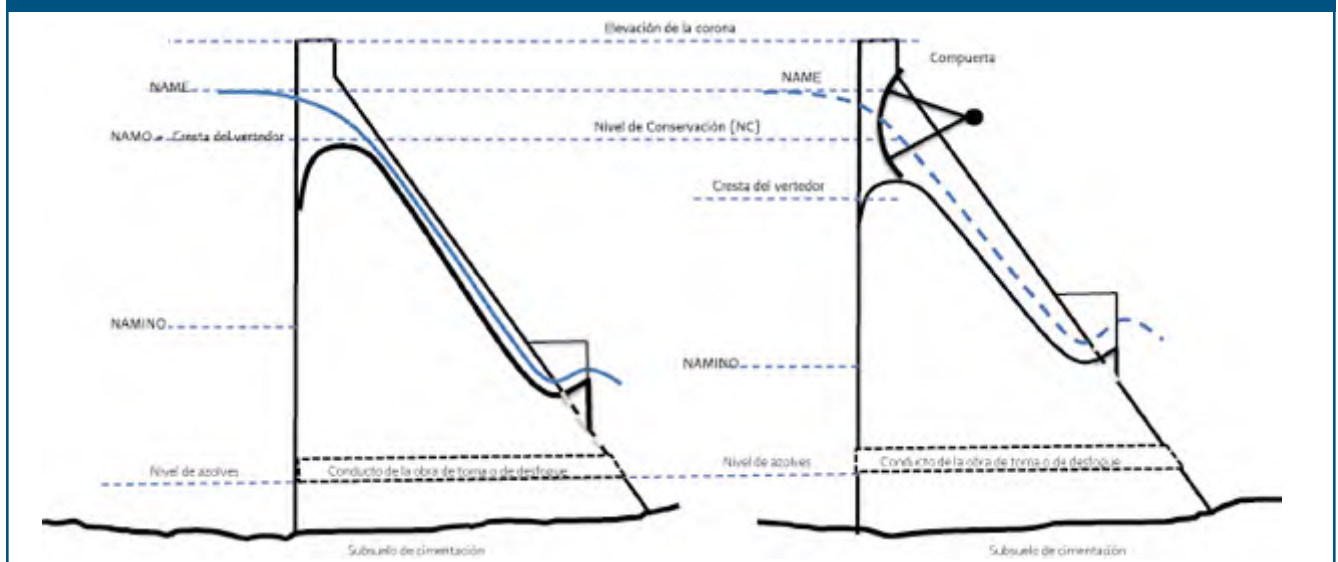
Figura 1. Conceptos de vertedores de excedencias libres y controlados
