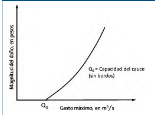
Figura 14. Relación Q_{\text{diseño}} - Magnitud del daño
