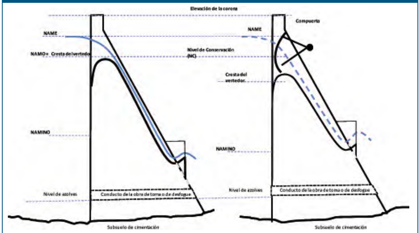
Figura 1. Niveles de almacenamiento en presas
