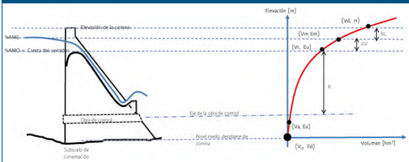
Figura 3. Presa de control de inundaciones y su curva embalse-capacidades
