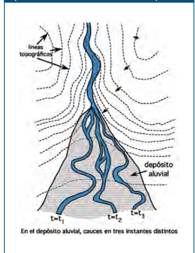
Figura 3.4. Inestabilidad natural en el depósito aluvial típico al salir de una zona encañonada a una planicie
