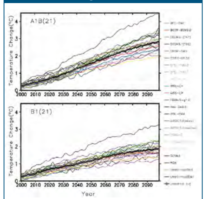
Figura 4. Evolución del cambio en la temperatura superficial del aire proyectada, promedio global, por 21 modelos distintos para dos escenarios (A1B y B1) moderados del IPCC (Fuente: IPCC, 2007, Fig.10.5)
