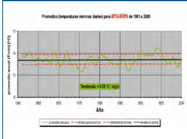
Figura 9. Tendencia promedio nacional en la temperatura mínima diaria: +0.08°C/siglo
