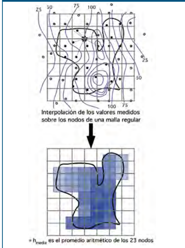
Figura 2.1.4. Método a través de interpolación a malla regular
