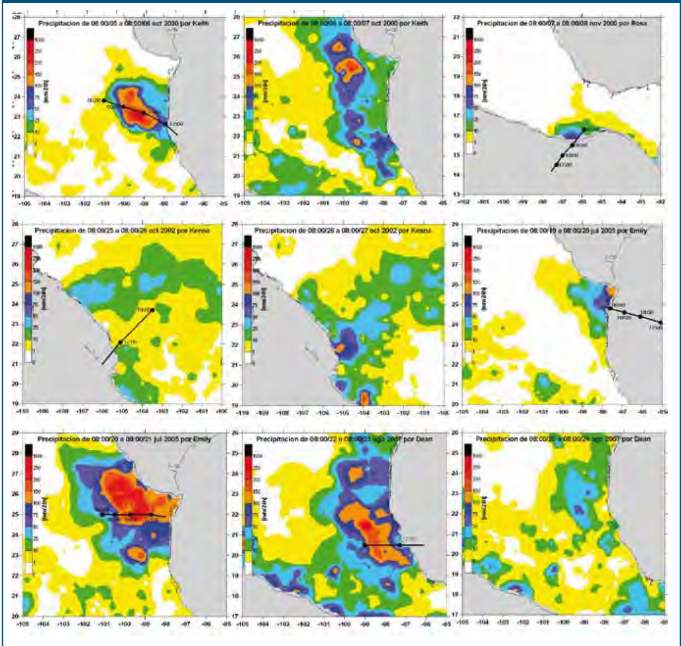
Figura 7. Huellas de precipitación de los ciclones tropicales Keith (2000), Rosa (2000), Kenna (2002), Emily (2005) y Dean (2007) incidiendo al continente en forma casi perpendicular, incluyendo algunos de los días en que estaban ya en estado de disipación (sin trayectoria sobrepuesta)
