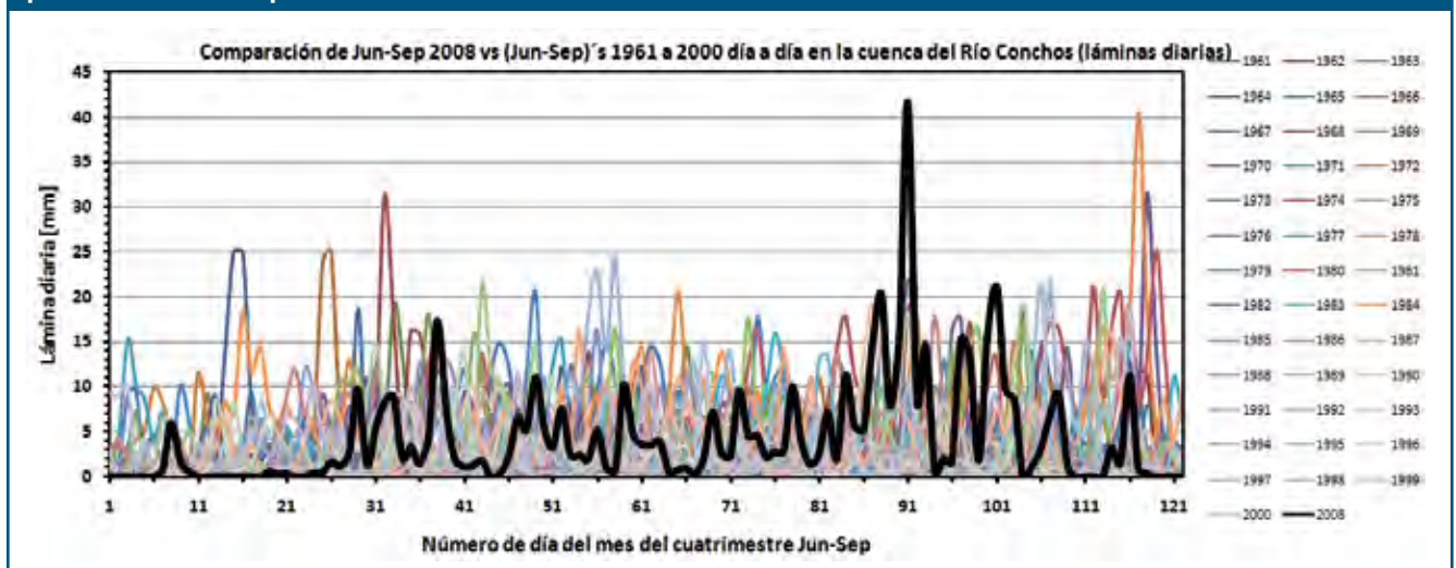
Figura 1.2.1.A-1. Trazas de las lluvias diarias de junio 1° a septiembre 30 para una muestra histórica 1961-2000 y para 2008, láminas promedio en la cuenca del río Conchos a su desembocadura al río Bravo
