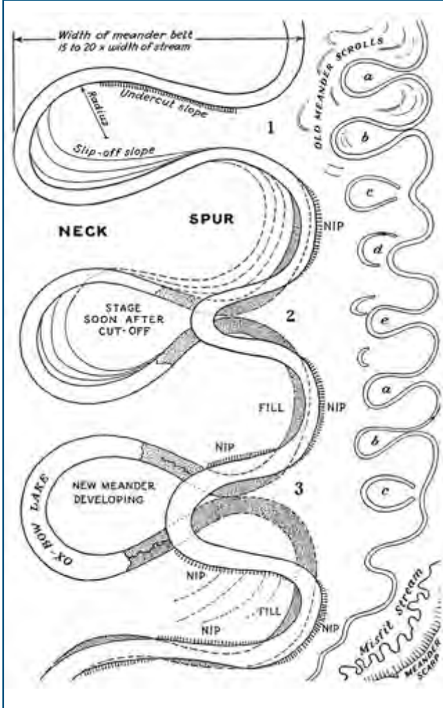
Figura 7. Desarrollo de un flujo meándrico en planicie aluvial en la cuenca baja
