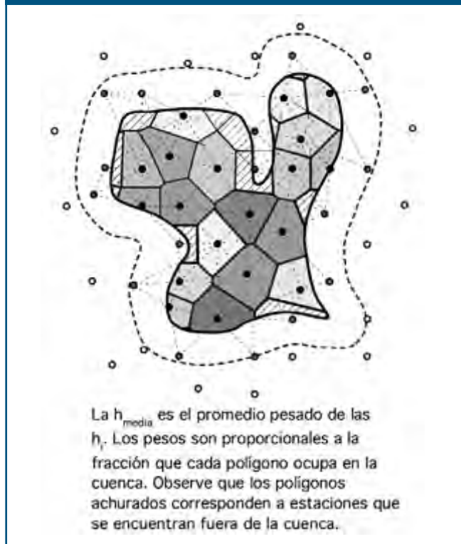
Figura 2.1.2. Método de polígonos de Thiessen
