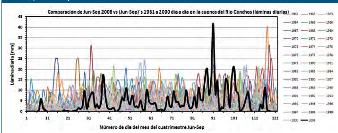
Figura 1.2.1.A- 2. Cuarenta registros cuatrimestrales de lluvias diarias, del 1° de enero (día 1) al 30 de septiembre (día 122) para las temporadas de lluvias 1961 hasta 2000
