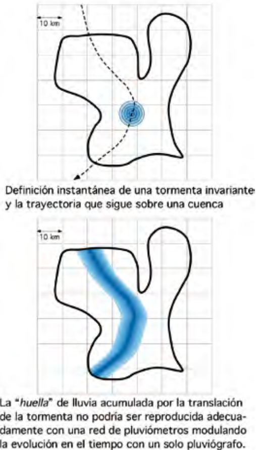
Figura 2.1.6. Variación temporal de la lluvia por translación de la tormenta
