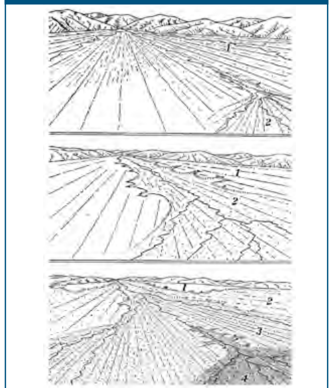
Figura 5. Etapas de desarrollo de un abanico aluvial
