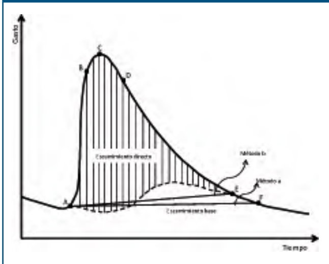
Figura 5. Separación del escurrimiento base del directo
