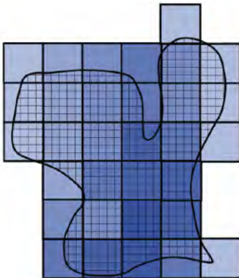
Figura 2.1.7. Celdas de un modelo lluvia escurrimiento, de un tamaño tal que las celdas de la evaluación de lluvia resultan múltiples exactos de ellas (5x5 a 1 en el ejemplo)
