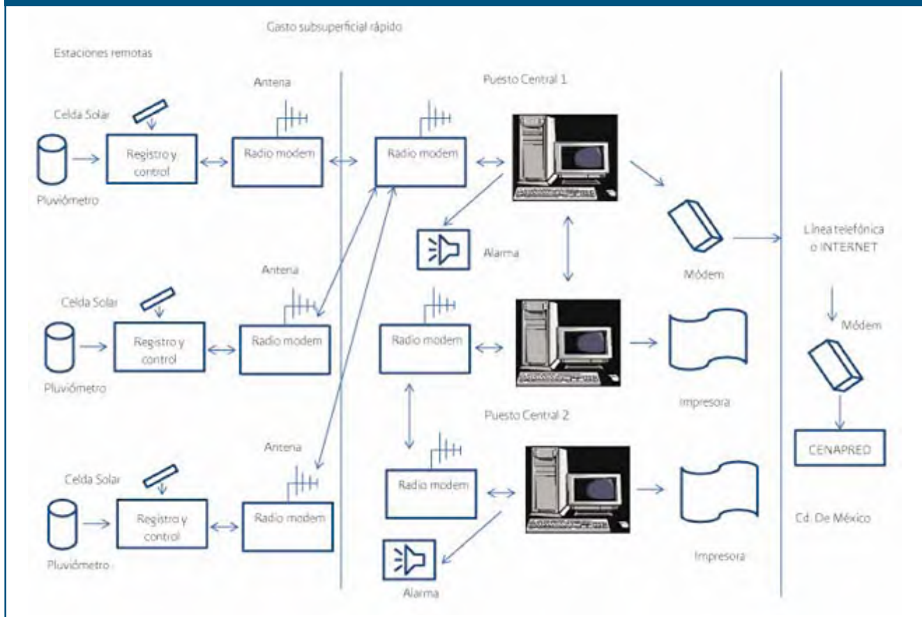
Figura 7. Diagrama general de un Sistema de Alerta Hidrometeorológica del CENAPRED
