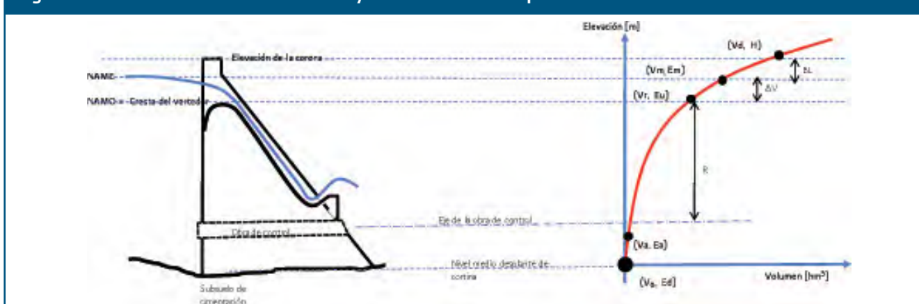
Figura 3. Presa de control de inundaciones y su curva embalse-capacidades
