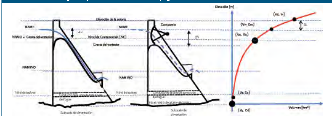
Figura 2. Curva elevaciones-capacidades del vertedor. Representación gráfica de los volúmenes de almacenamiento de agua respecto a las elevaciones topográficas del embalse
