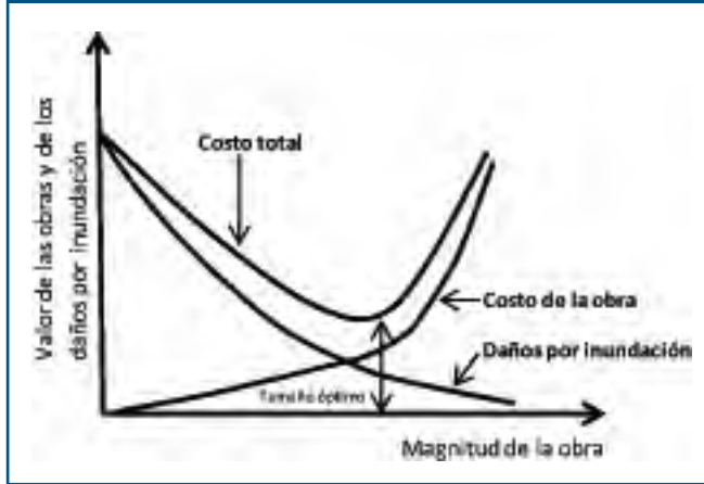
Figura 13. Selección de la magnitud óptima de una obra de protección
