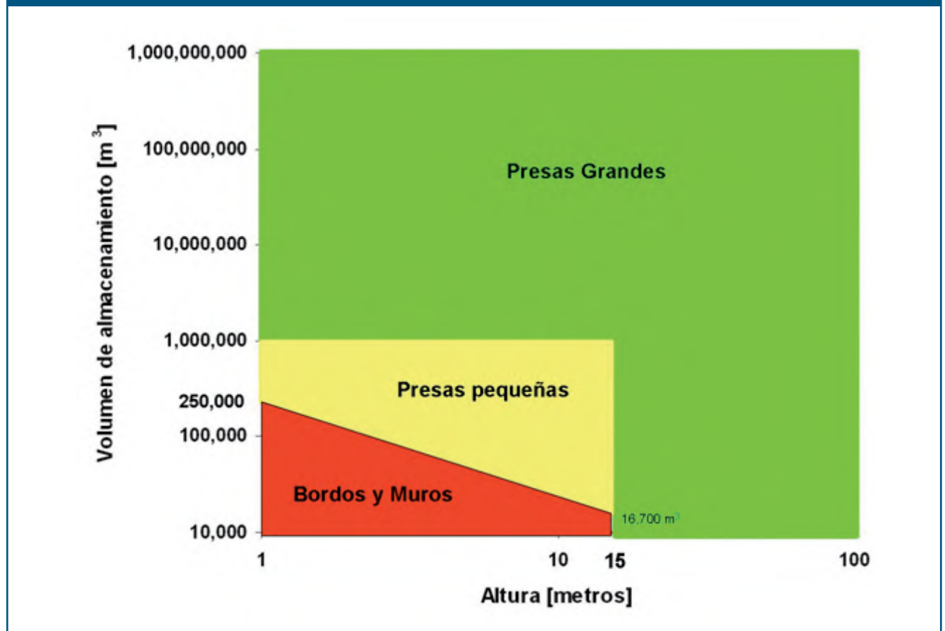
Figura 1. Tamaño de presas
