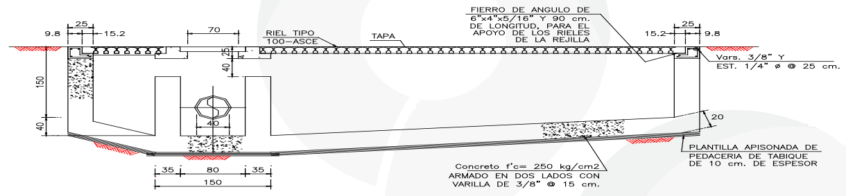
C O R T E D - D ACOT. CM ESC. SIN
