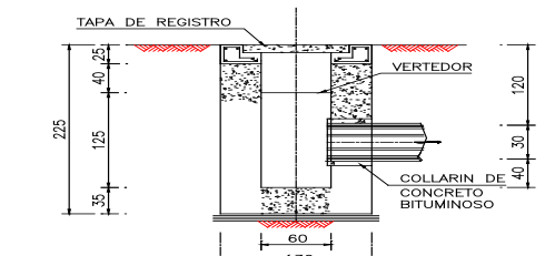
C O R T E E - E ACOT. CM ESC. SIN
