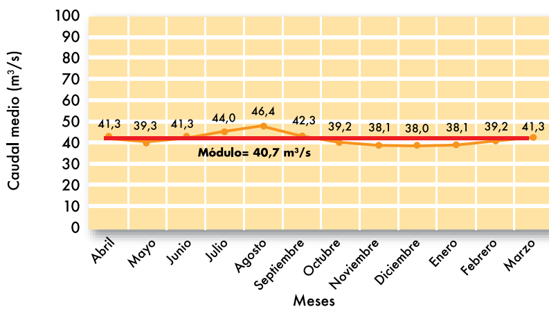
Hidrograma de caudales medios mensuales (Serie 1992-2009) río Chubut en Valle Inferior
