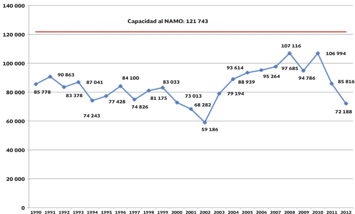
G4.1 Volumen en las 172 presas (hm 3 )
