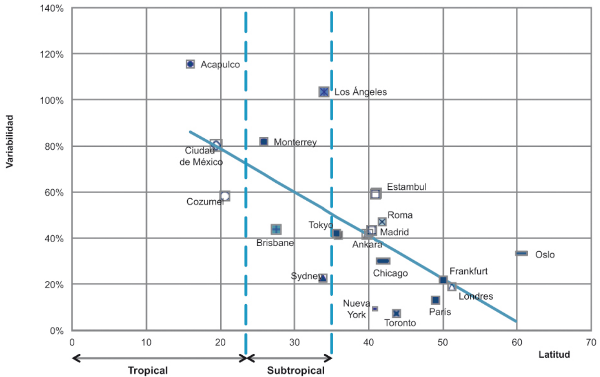
G8.3 Interrelación entre la variabilidad de la precipitación y latitud
