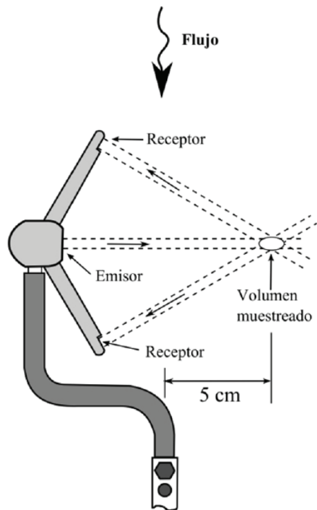
Figura 52. Diagrama del velocímetro acústico Doppler.
