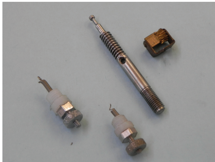
Figura 29. Componentes básicos de la cámara de contactos.
