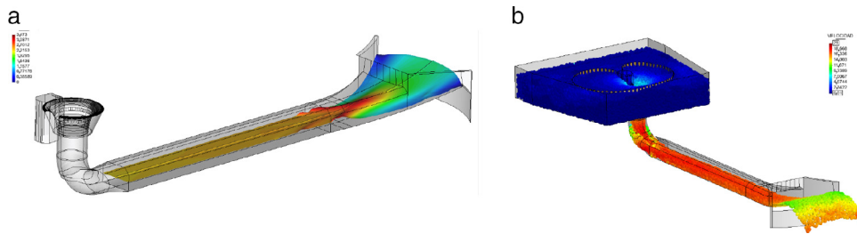
Figura 7. Caudal 378 m 3 /s. Nivel de embalse 590,87 msnm. Vo = 17,9 m/s. (a) Modelo Iber. (b) SPHERIMENTAL.
