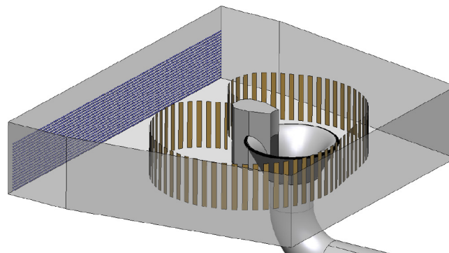
Figura 6. Límites del depósito de alimentación del modelo tridimensional y pantalla de tranquilización y uniformización del flujo de aproximación.
