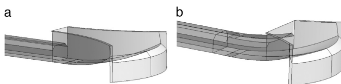
Figura 3. Estructura de disipación de energía en desembocadura. La figura b introduce un carrete de transición para aumentar la sección de salida al embalse de Itoiz.
