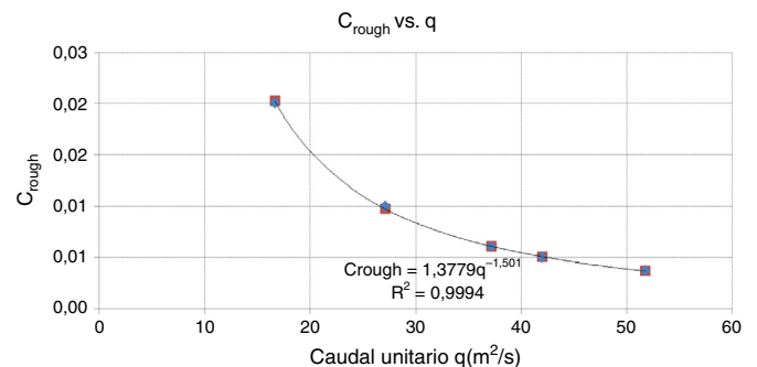
Figura 9. Caudal 378 m 3 /s. Nivel de embalse 590,87 msnm. Comparación de velocidad y lámina en el eje del canal de descarga entre ambos modelos. Iber (n = 0,016, vo = 17,9 m/s) y SPH (C rough = 0,005).
