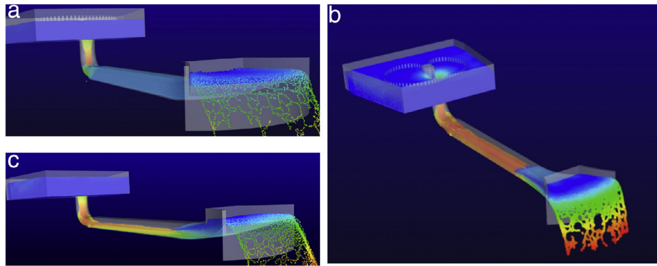
Figura 12. Funcionamiento del aliviadero para diferentes caudales.
