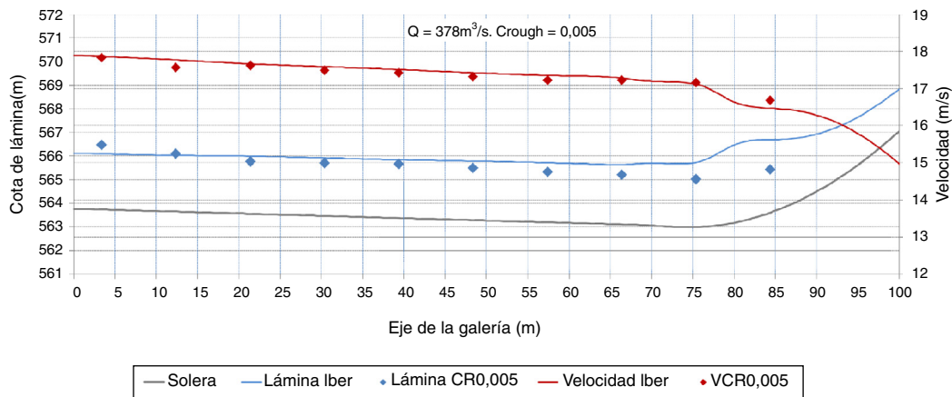
Figura 8. Caudal 378 m 3 /s. Nivel de embalse 590,87 msnm. Comparación de velocidad y lámina en el eje del canal de descarga entre ambos modelos. Iber (n = 0,016, vo = 17,9 m/s) y SPH (C rough = 0,005).
