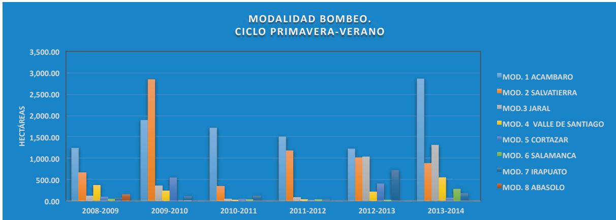
Gráfica 2.6 Superficie total regada por bombeo en el ciclo Primavera-Verano en cada uno de los módulos que conforman la zona de estudio
