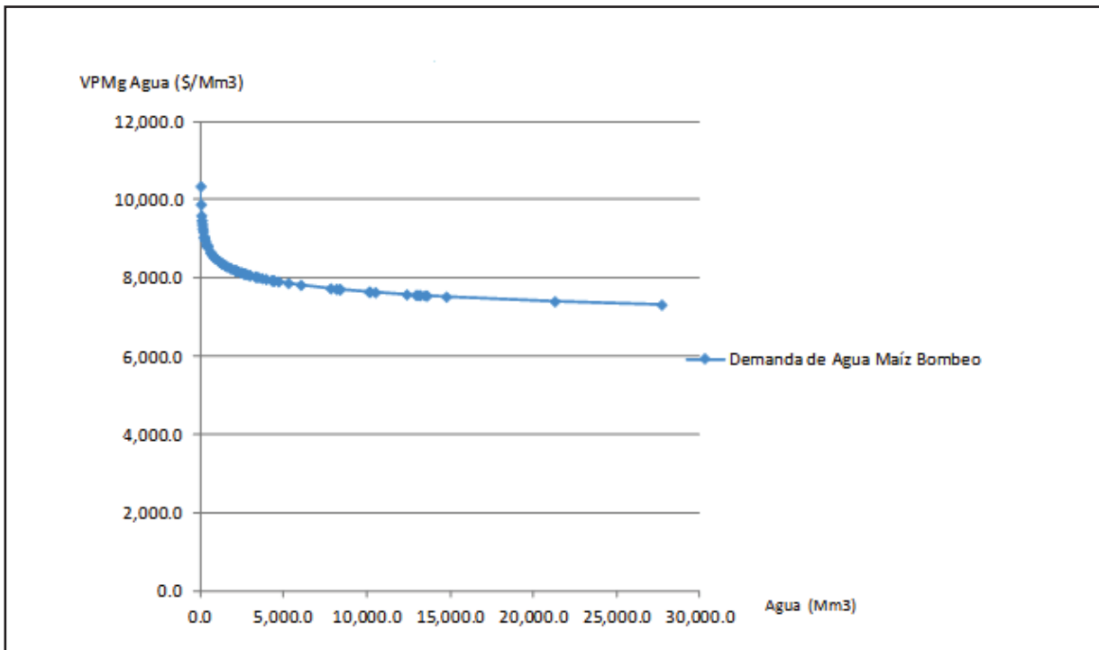
Gráfica 3.14 Función de demanda de agua de Maíz, con riego por bombeo
