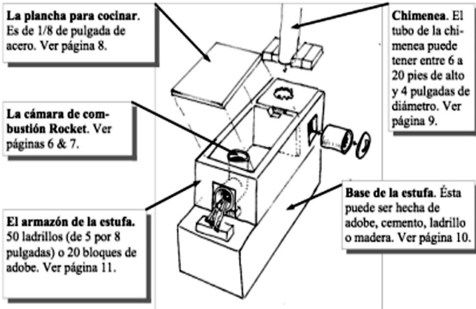
Prototipo de la empresa Aprovecho manufacturados a gran escala.
