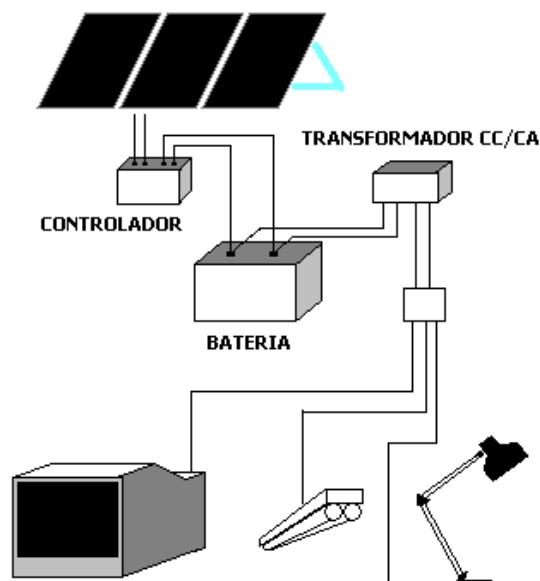
ESQUEMA SISTEMA AISLADO
