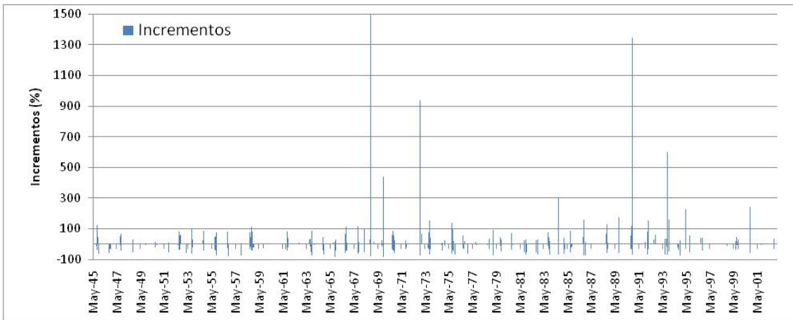
Figura 10. Tasa de cambio de los caudales diarios por evento de avenidas (1945-2002)
