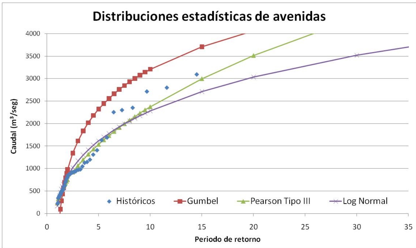
Figura 8. Distribuciones estadísticas para identificar la magnitud de las avenidas tipo a distintos periodos de retorno
