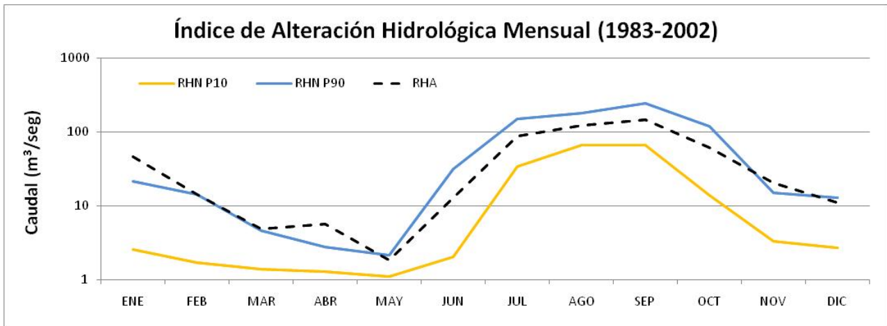
Figura 3. RHN VS RHA. Serie de aportación media mensual en escala logarítmica
