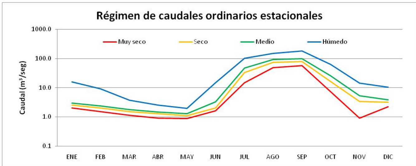
Figura 6. Representación gráfica de los regímenes hidrológicos para cada percentil representativo de distintas condiciones hidrológicas
