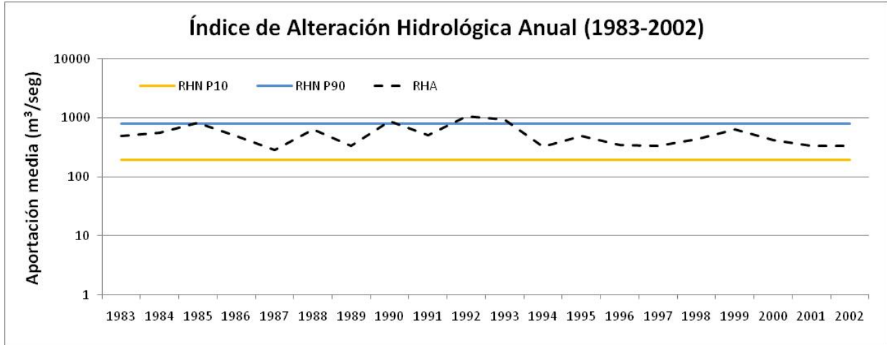
Figura 5. RHN VS RHA. Serie de aportación anual en escala logarítmica
