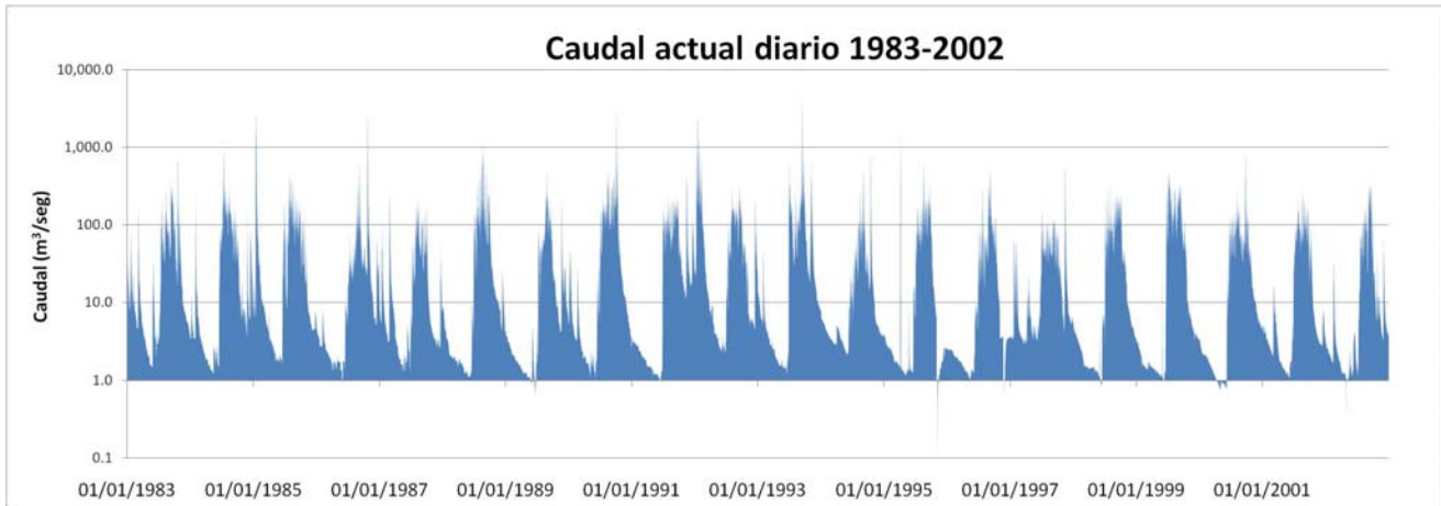
Figura 2. Representación gráfica de los regímenes diarios hidrológicos natural y actual en escala logarítmica
