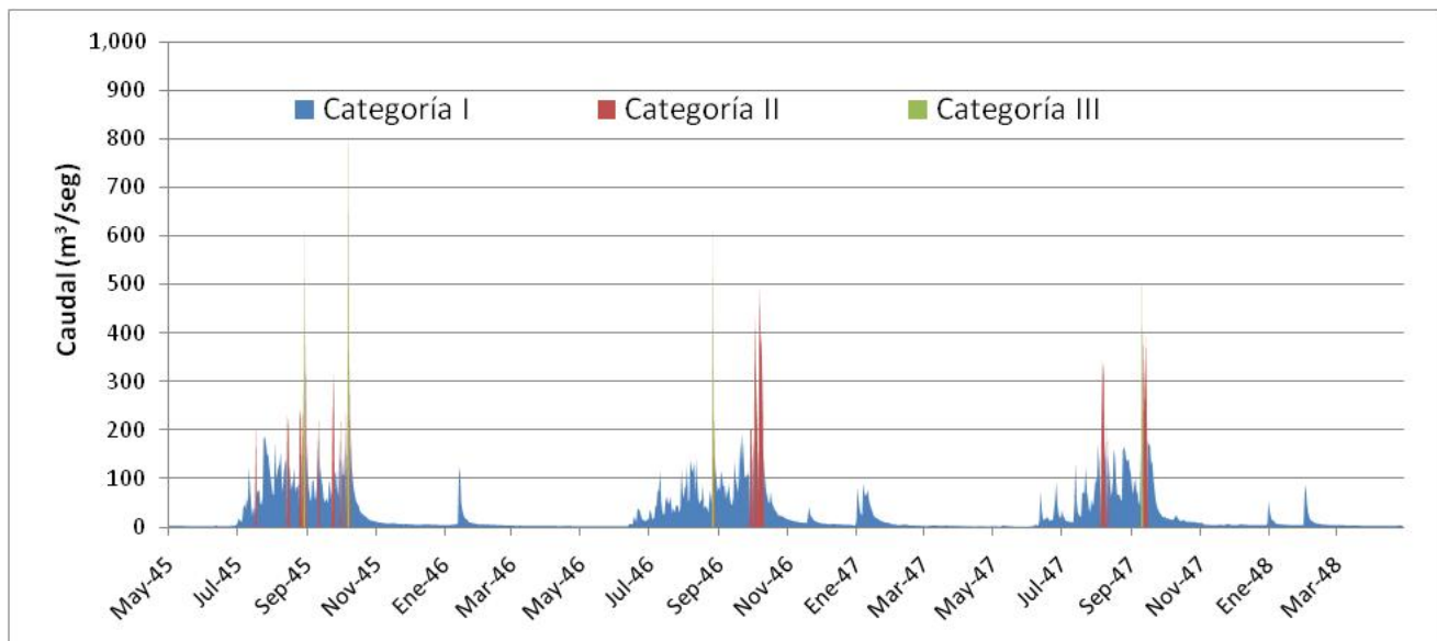
Figura 9. Caudales diarios identificados entre los umbrales de cada categoría en los años 1945-1948
