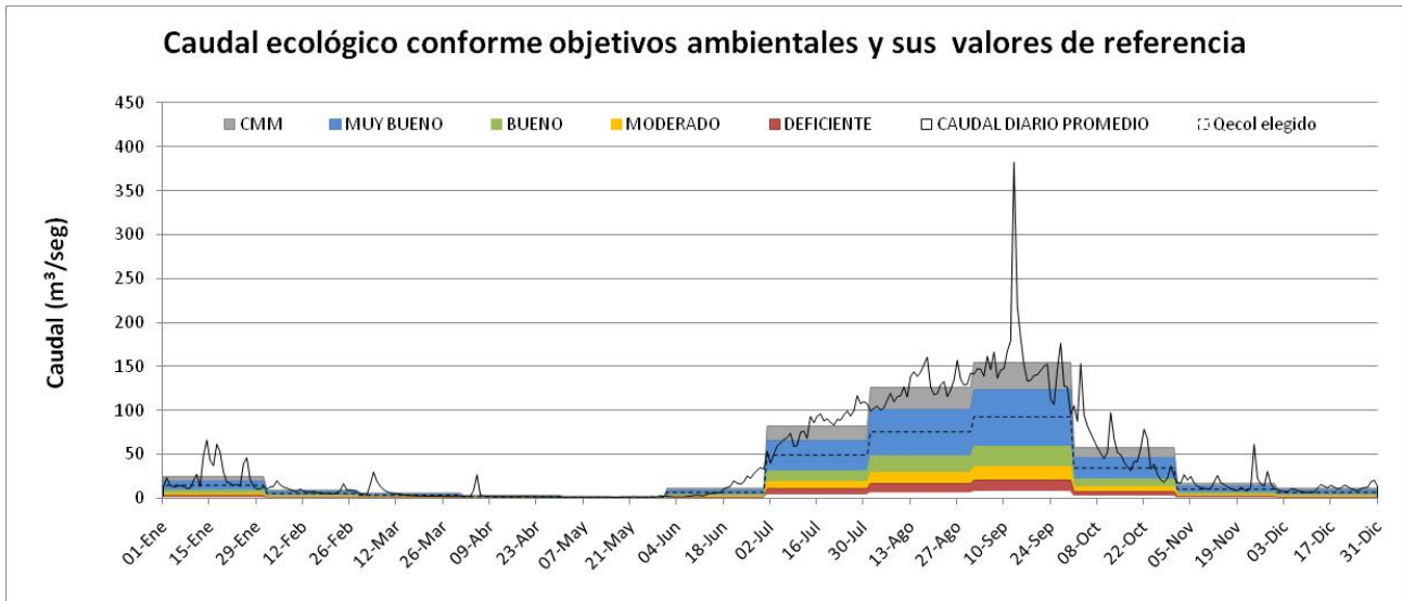
Figura 1. Régimen de caudal ecológico para el ejemplo del río Acaponeta (corriente permanente - unidades en m 3 /seg)
