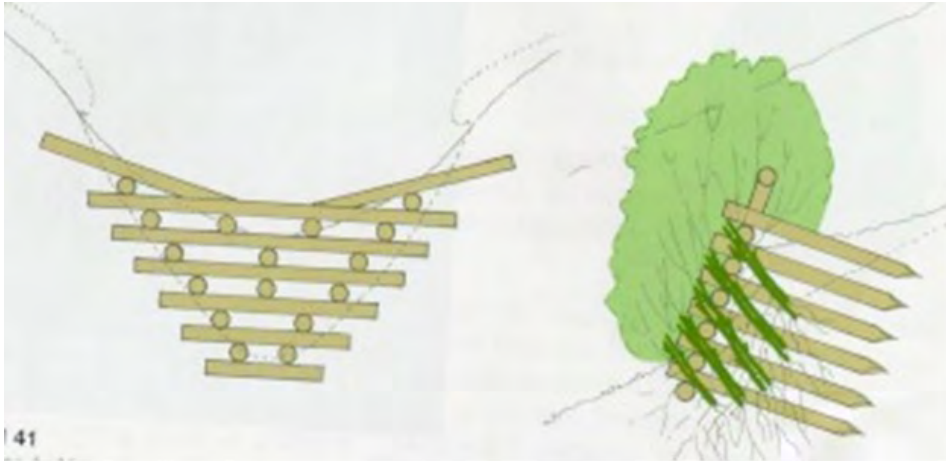
Figura 3.5.3. Colocación de represas filtrantes con estacas retoñable fuente: schiechl y stern, 2001, abb. 41
