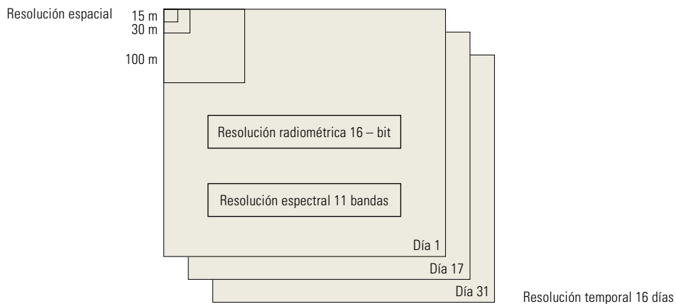
FIGURA 7.12 Resoluciones de una imagen de satélite Landsat 8 OLI-TIR. (Modificado de ERDAS 1997).
