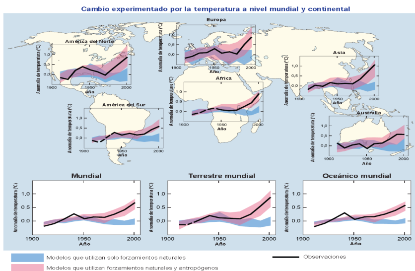
Figura 3. Incremento observado de la temperatura mundial respecto del promedio del periodo 1901-1950 (IPCC, 2007).
