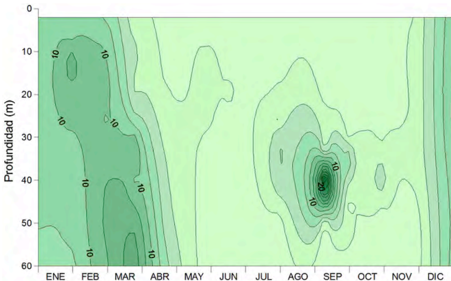
Figura 5.8. Dinámica anual de la concentración de la clorofila-a (en mg m -3 ) de la columna de agua del lago Alchichica. (Figura: José Daniel Cuevas Lara y Luis A. Oseguera Pérez).
