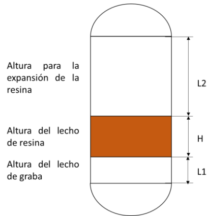
Fig. 1- Variables que forman parte del dimensionamiento del ablandador
