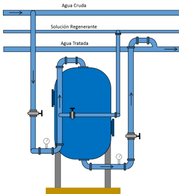
Fig. 2- Ablandador tipo de la Planta de tratamiento de agua de la Refinería de petróleo Níco López
