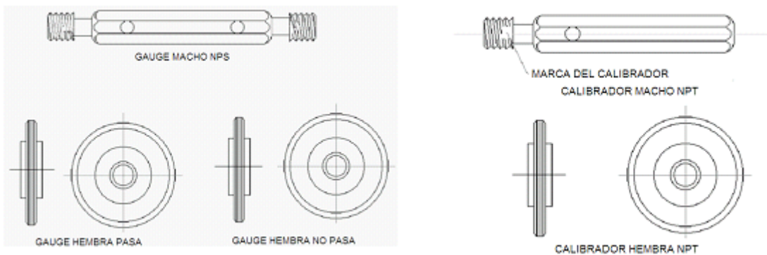
Figura 1.- Calibrador maestro macho o hembra
