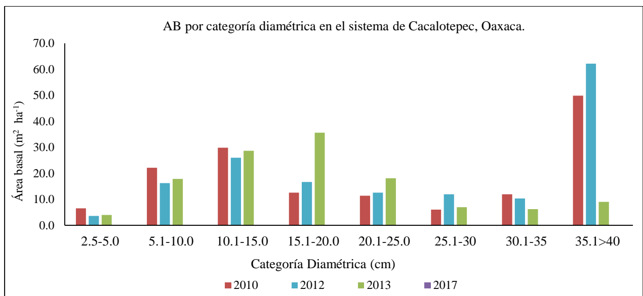
Gráfica 74. Área basal por categorías diamétricas en el sistema Cacalotepec, Oaxaca.
