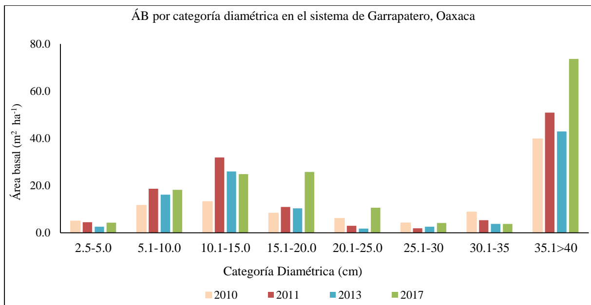
Gráfica 47. Área basal por categoría diamétrica en el sistema Garrapatero, Oaxaca.
