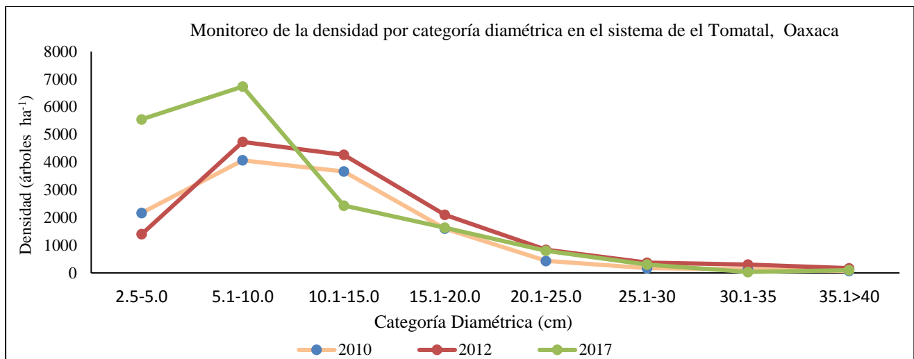
Gráfica 66. Registro de la densidad del arbolado en el sistema lagunar El Tomatal, Oaxaca.
