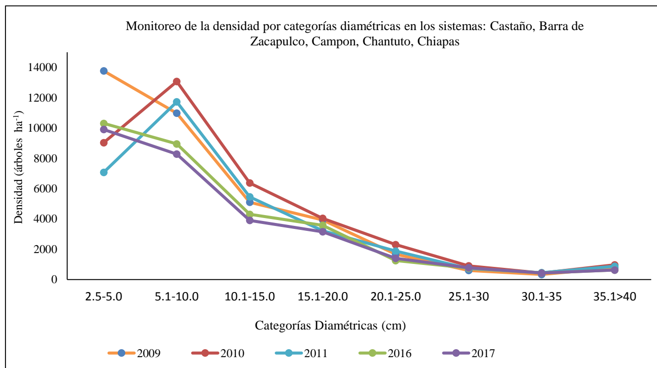
Gráfica 18. Monitoreo de la densidad del arbolado en los sistemas: Castaño, Barra de Zacapulco, Campón, Chantuto, Chiapas
