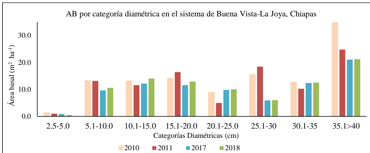
Gráfica 32. Distribución del área basal por categorías diamétricas en el sistema Buenavista-La Joya, Chiapas.
