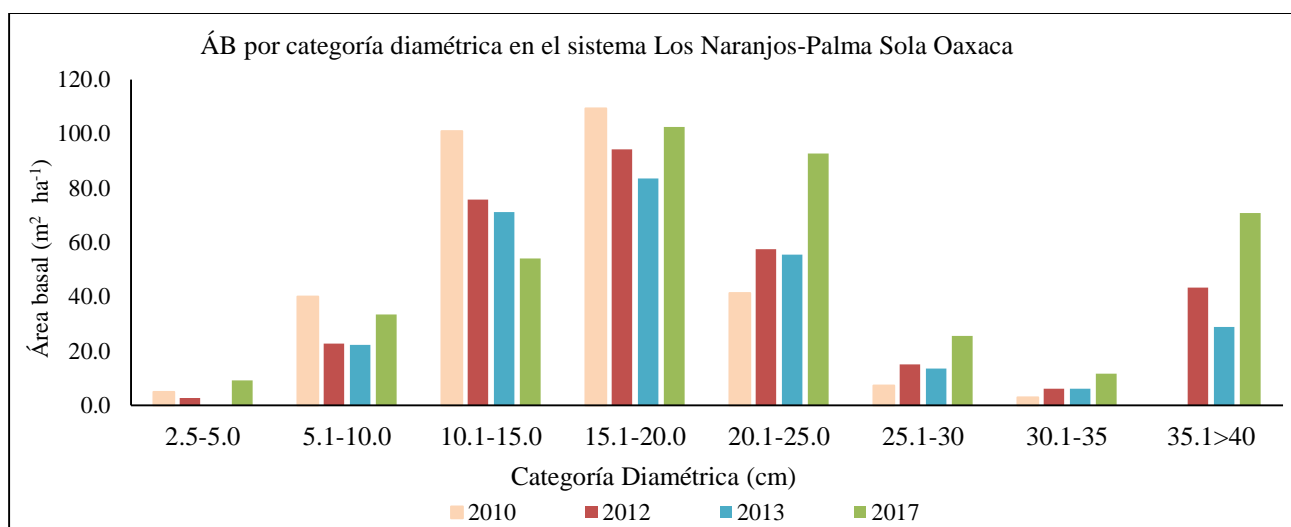
Gráfica 68. Área basal por categoría diamétrica en el sistema Los Naranjos-Palma Sola, Oaxaca.
