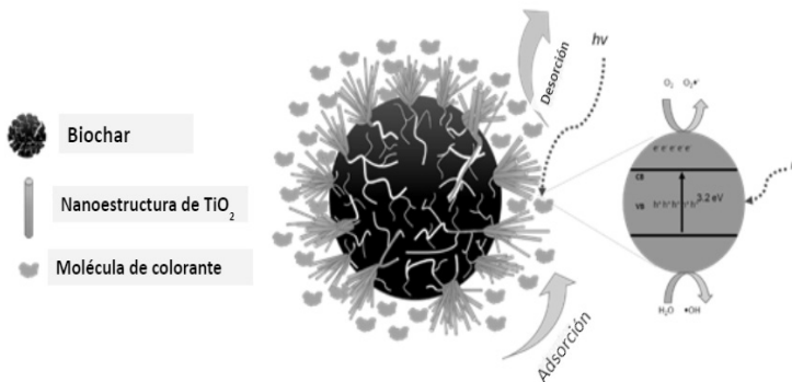
Figura 2. Efecto sinérgico de compuesto a base biochar con nanopartículas 1-D de \text{TiO}_2
