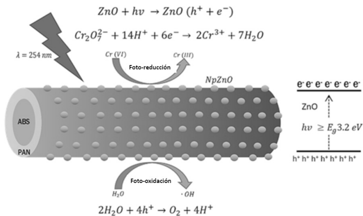
Figura 3. Esquema catalítico de la fotoreducción de Cr (VI), mediante nanopartículas de ZnO embebidas en fibras poliméricas coaxiales compuestas por ABS/PAN
