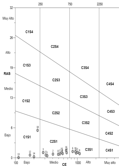
Figura 4. Clasificación del agua de acuerdo a la CE vs RAS, para los valores promedio del acuífero Alto Atoyac
