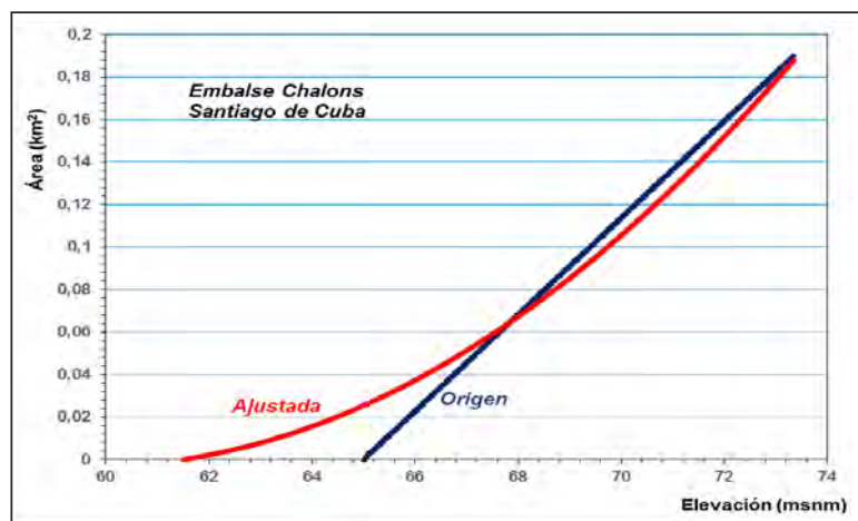
Figura 5-1. Curvas típicas de Área VS Elevación del embalse Chalons, provincia Santiago de Cuba (106 años)
