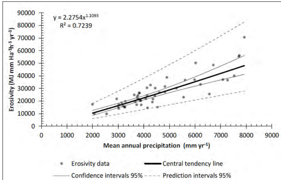
Figura 4-5. Factor R como función de la precipitación media anual
