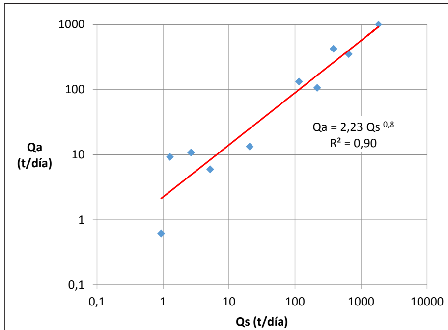
Figura 2-6. Relación entre el sedimento de arrastre ( Q_a ) y el sedimento en suspensión ( Q_s ) en el río Areias, Brasil
