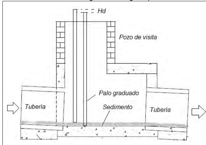
Figura 2-14. Sección de una galería de aguas pluviales monitoreada
