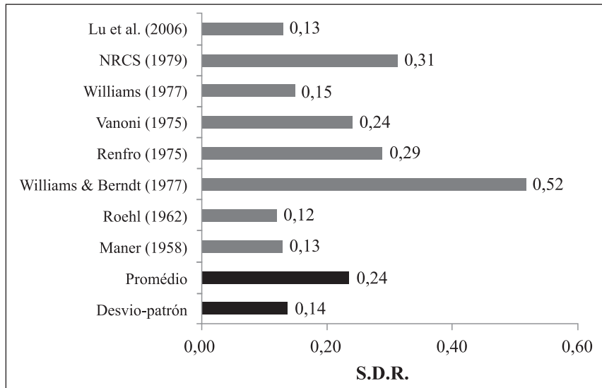
Figura 2-5. Valores de SDR calculados para la cuenca del río Pípiripau (DF), utilizando 8 ecuaciones distintas
