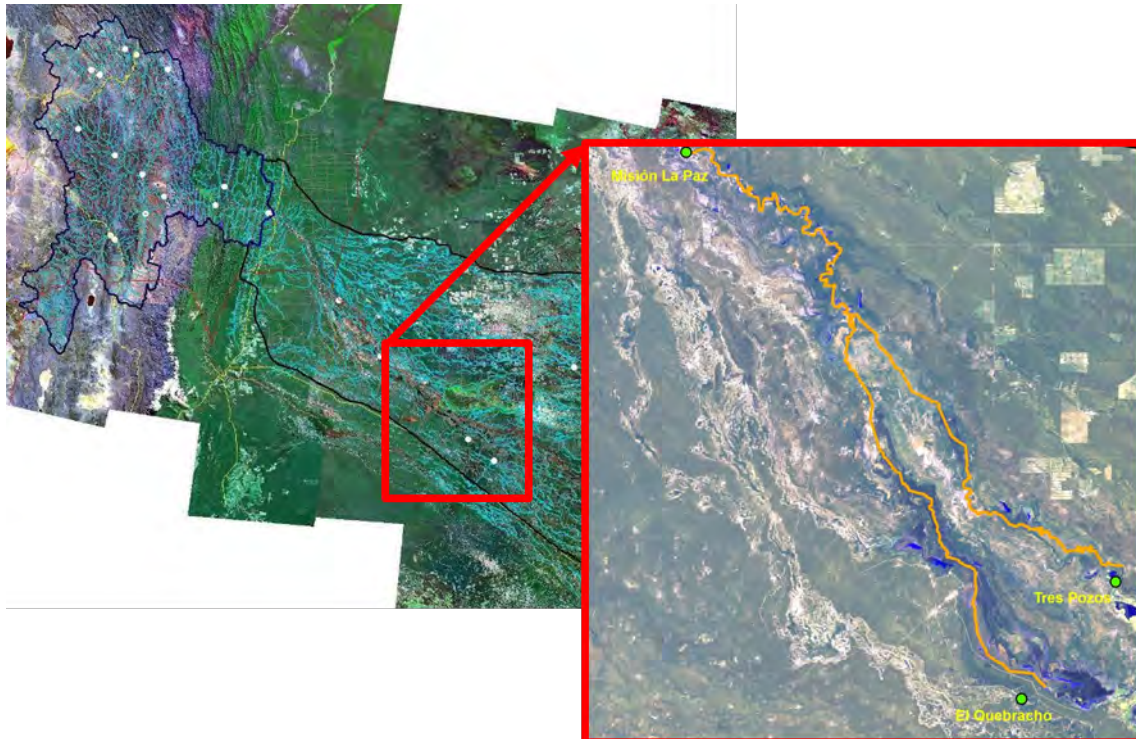
Figura 1-8. Bifurcación del río Pilcomayo en el “Pantalón”
