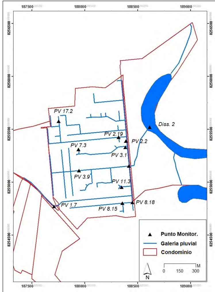
Figura 2-15. Galerías pluviales en el Condominio Noroeste (Brasília-DF), con los puntos de monitoreo de S c
