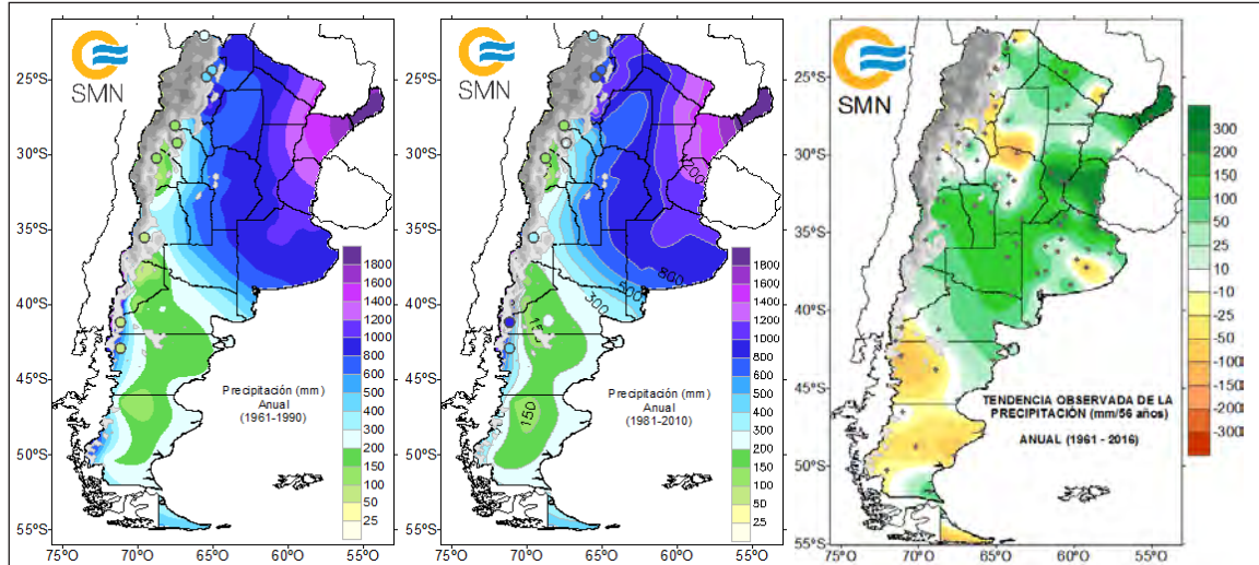
Figura 1-1. Precipitación media anual períodos 1961-1990 y 1981-2010, y tendencias de cambio de la precipitación
