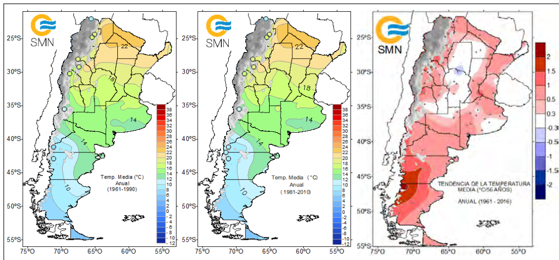
Figura 1-2. Temperatura media anual períodos 1961-1990 y 1981-2010, y tendencias de cambio de la temperatura media
