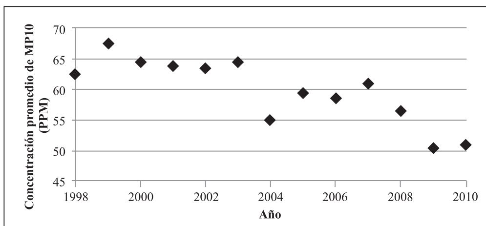
Figura 6-3. Evolución de la concentración de MP10 en 279 ciudades estadounidenses tras la creación de la normativa de control de sedimentos
