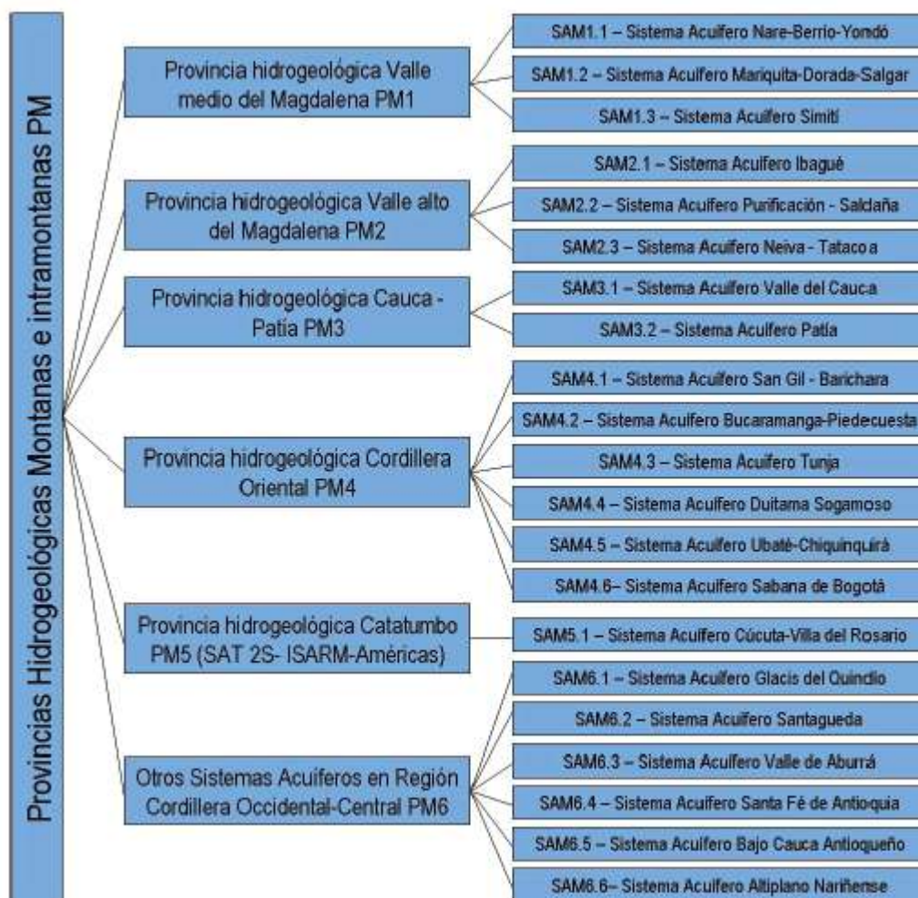
Figura 8. Sistemas acuíferos de las provincias hidrogeológicas montanas e intramontanas
