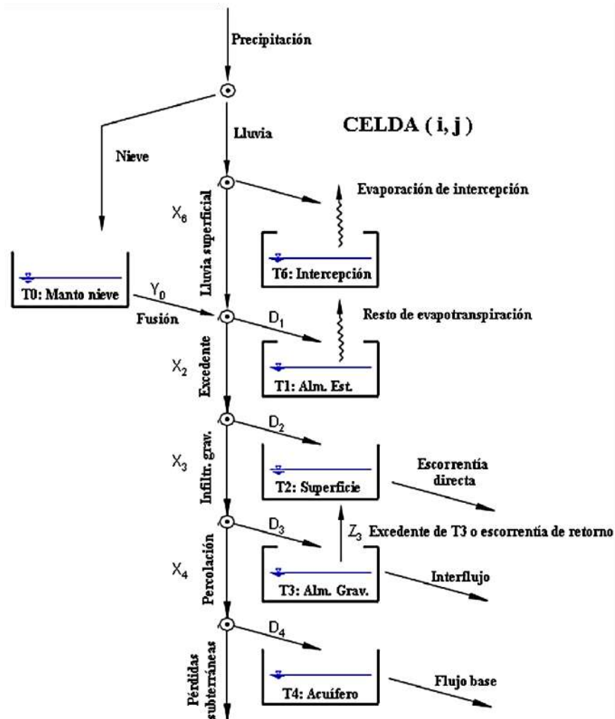
Figura 10. Esquema conceptual de tanques a nivel de celda del modelo TETIS.
