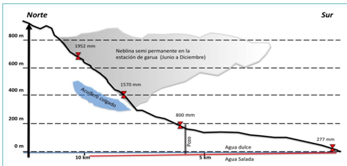
Figura 2. Modelo hidrogeológico en la parte barlovento de la isla Santa Cruz (la presencia del acuífero colgado aún no se ha confirmado). El diagrama fue interpretado de los estudios de Percy, et al. 2016, Pryet, et al. 2012 y de los estudios de GIIWS
