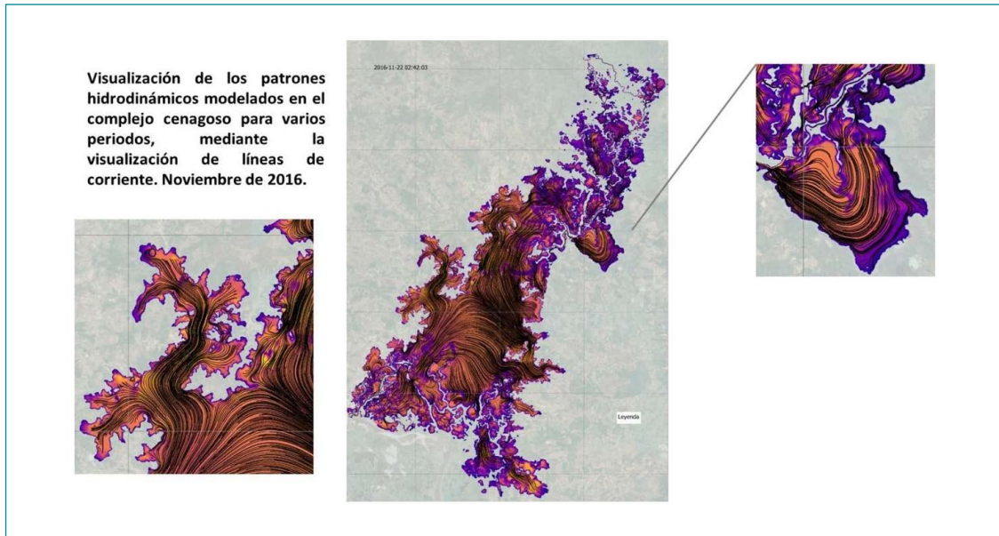
Figura 9. Modelos Hidrodinámicos: Sitio demostrativo ECH – CCZapatososa.
